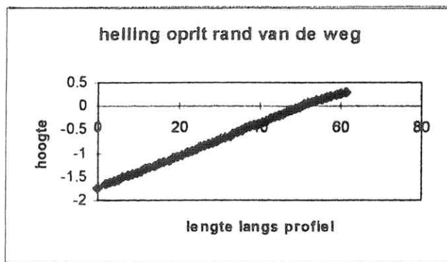
Figuur 3 : profiel rand van de weg
