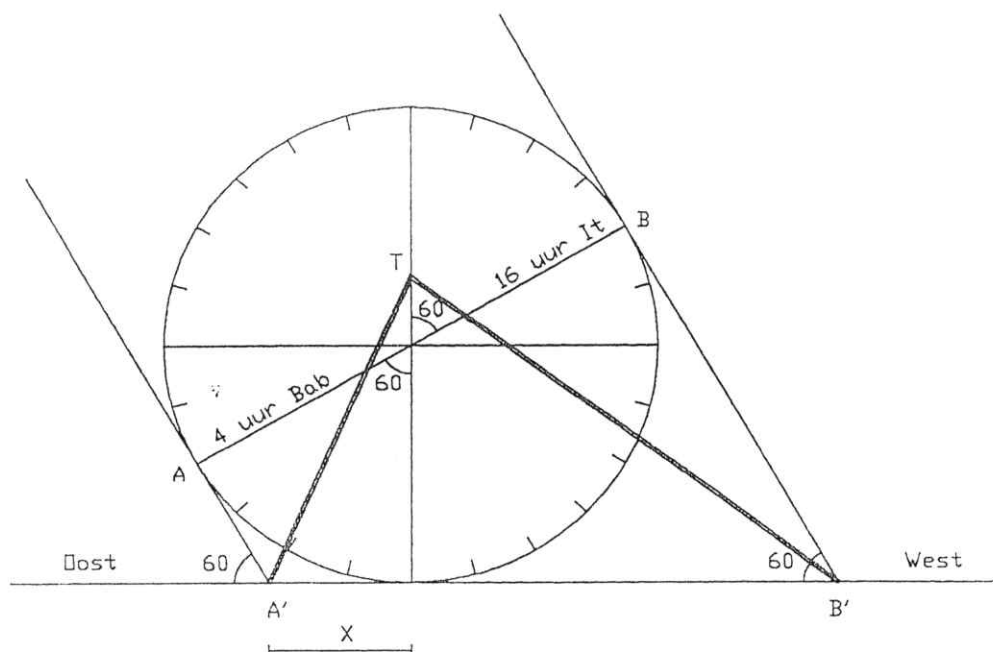
Figuur 2 : Constructie van de uurlijnen
